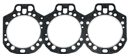
56111903 - DIÂMENTRO 133 MM
