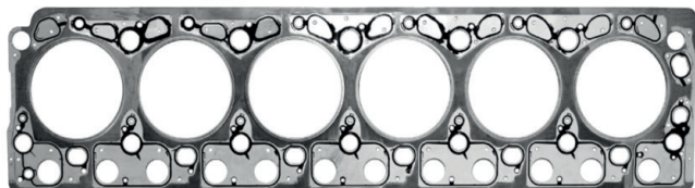
56182105 - DIÂMETRO 103,7 MM
