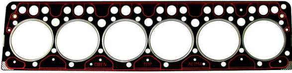
56149603-DIÂMETRO 98.5MM
